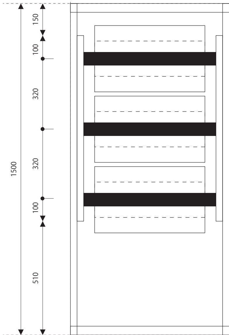
正面図
