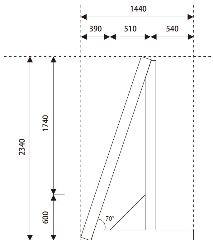
側面図
