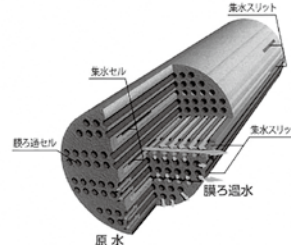
● 膜エレメントの構造
