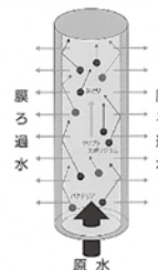
● 内圧全量ろ過方式のしくみ
