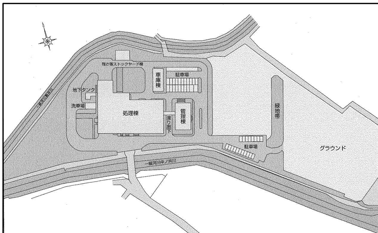
図3.2.4 施設配置図
