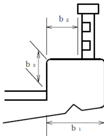
图 3-13 地覆寸法
