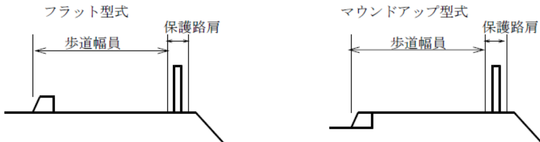
図 3-11 歩道の形式
