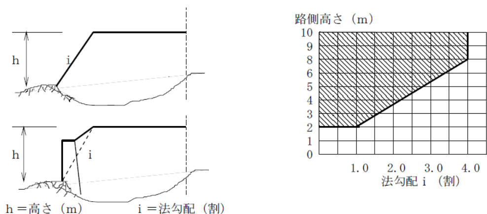
図 3-15 法勾配と路側高さの関係
