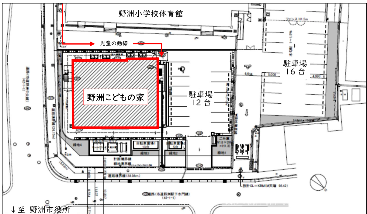
(配置図)
