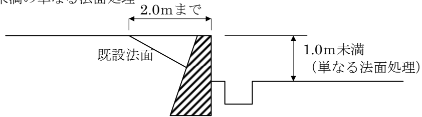
例1 1m未満の単なる法面処理
