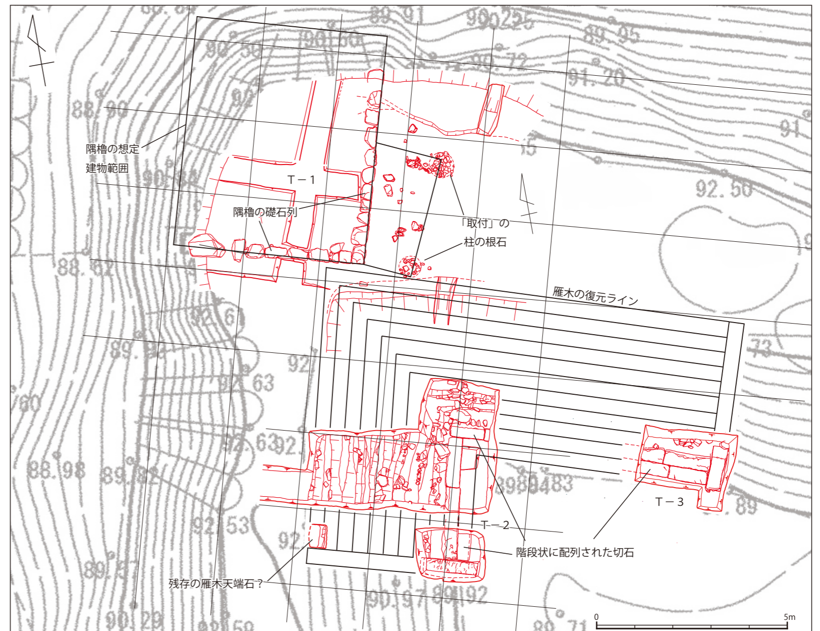
史跡永原御殿跡 令和4年度発掘調査区 (本丸「乾角御矢倉」) 遺構平面図
