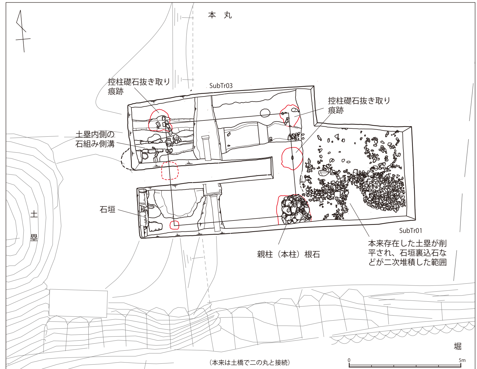
永原御殿跡 令和2年度調査区 遺構平面図
