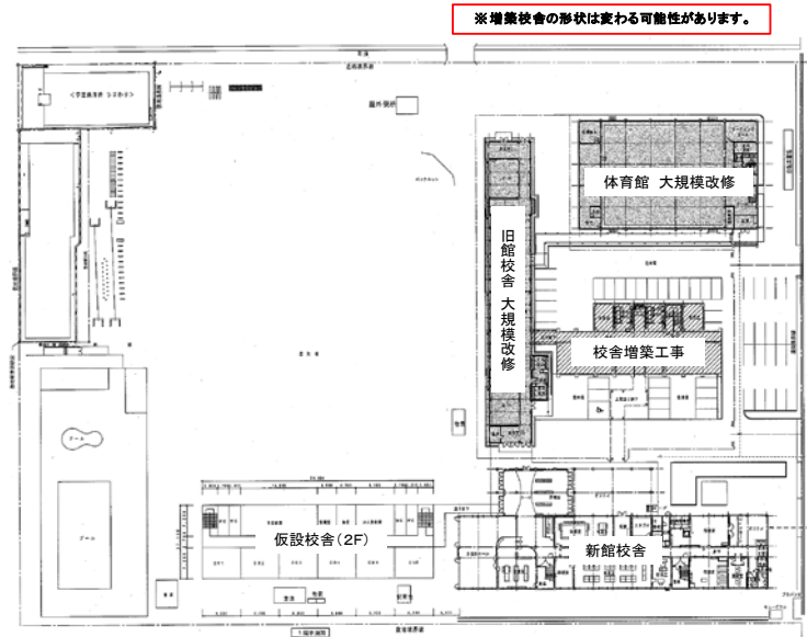
平成31年10月 ~ 平成32年12月 敷地内配置図
